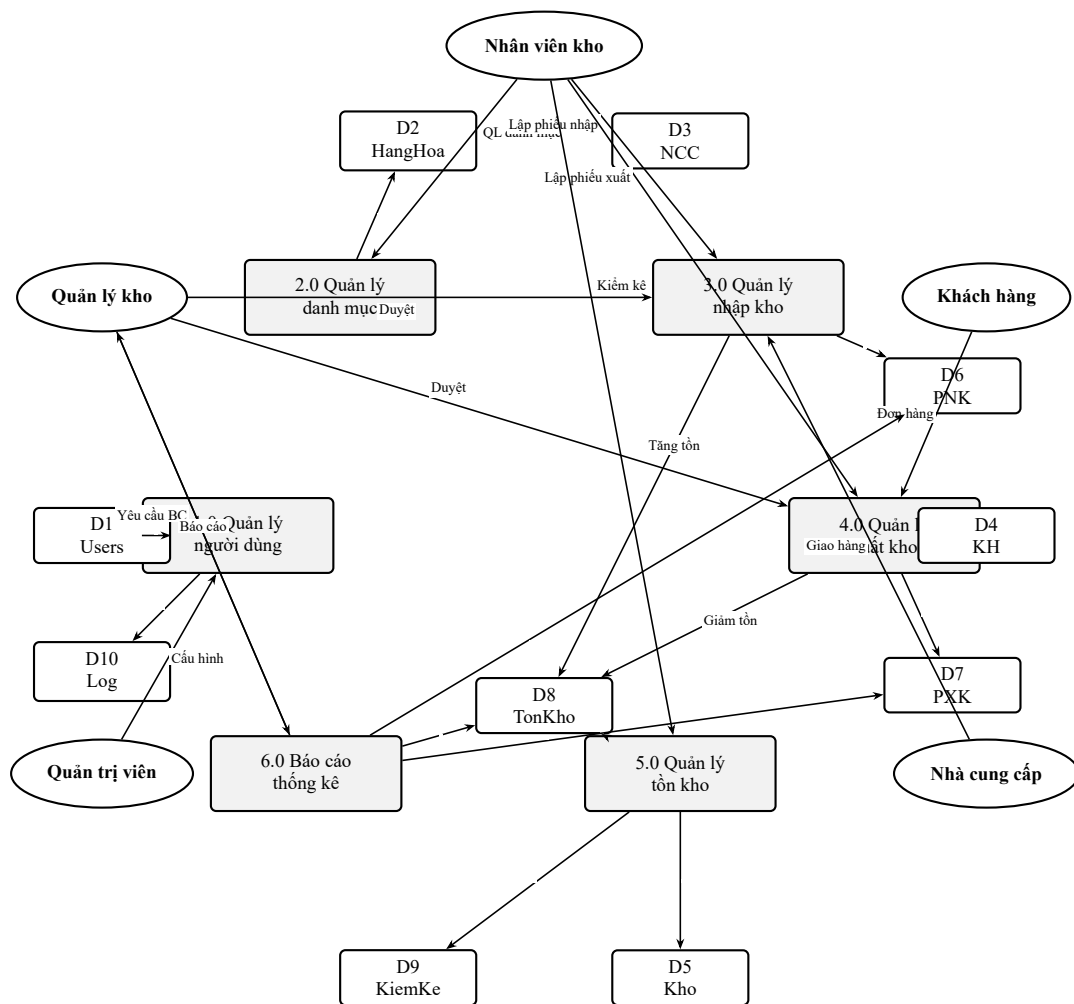
Hình 1: DFD cấp 1 – Phân rã các luồng dữ liệu trong hệ thống quản lý kho hàng
